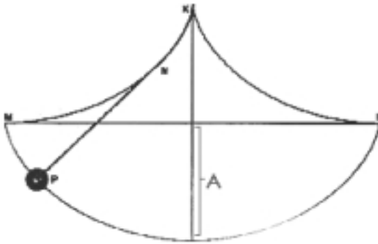
Cycloidal pendulum.
